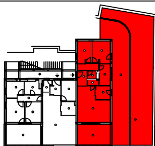
TLOCRT PRIZEMLJA
